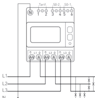
3 PHASEN - 4 LEITER
