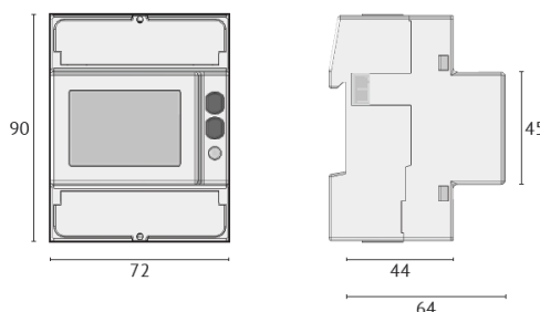
Abmessungen (mm):
