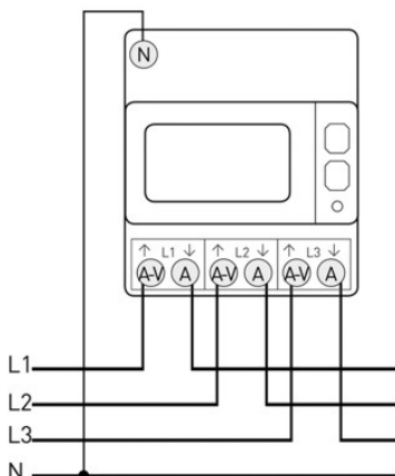
3 Phasen - 4 Leiter
